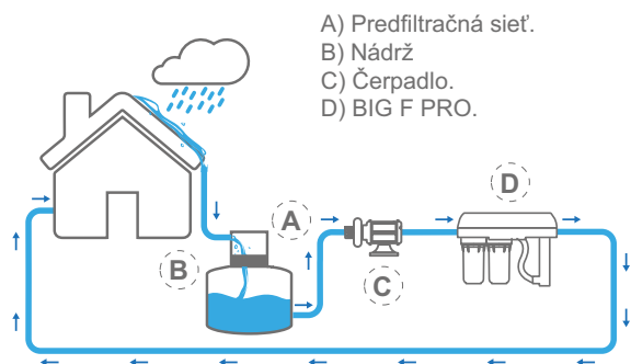
1 Úprava dažďovej vody
